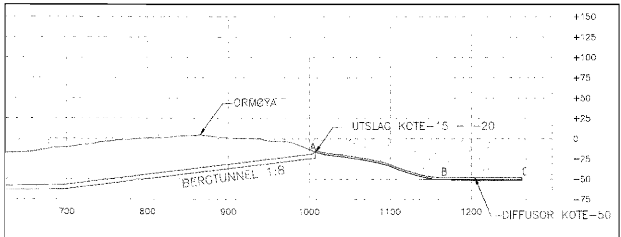
Fig 2: Lengdesnitt av utslippstunnel og utslippsledning
